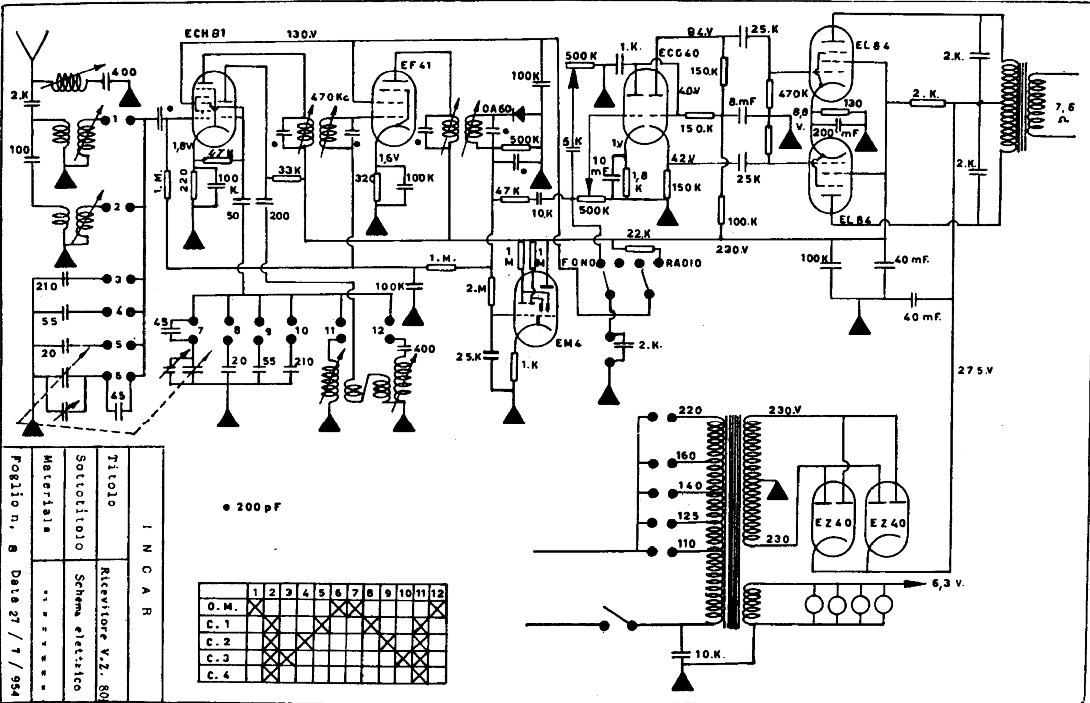
INCAR.. Mod. VZ 803. Ricevitore a onde medie con quattro bande allargate in onde corte. Potenza d'uscita 8 watt. Consumo 90 watt.
